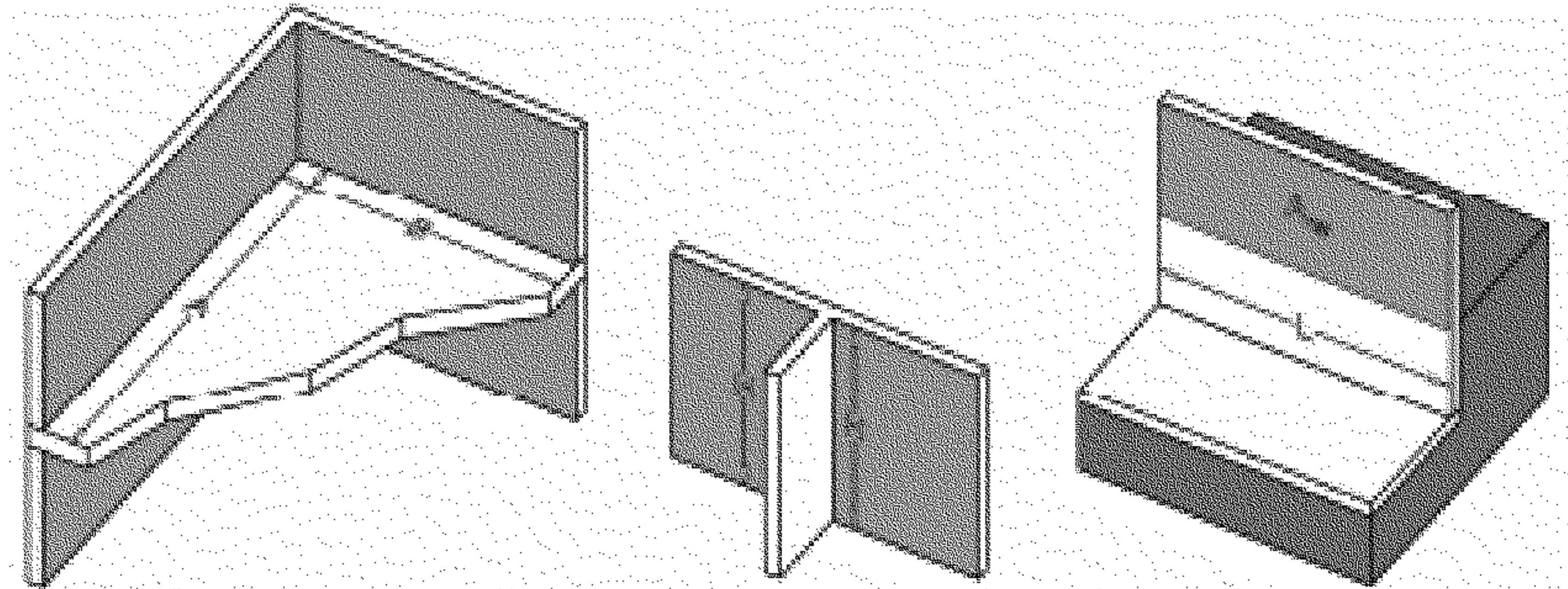
پل حرارتی دیوار مجاور پل حرارتی تقاطع دیوارهای پل حرارتی کف بین طبقات: خاک: L داخلی و خارجی: 2 \times H 2 \times (A+B)
